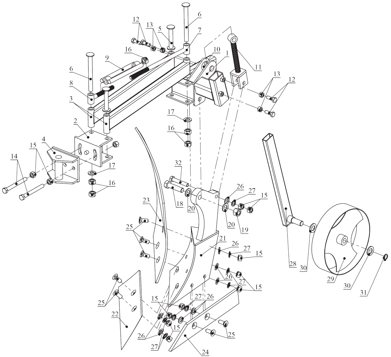
Рисунок 4. Комплектующие навесного плуга PL-130.
