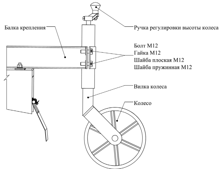
Рисунок 9. Установка колеса.
