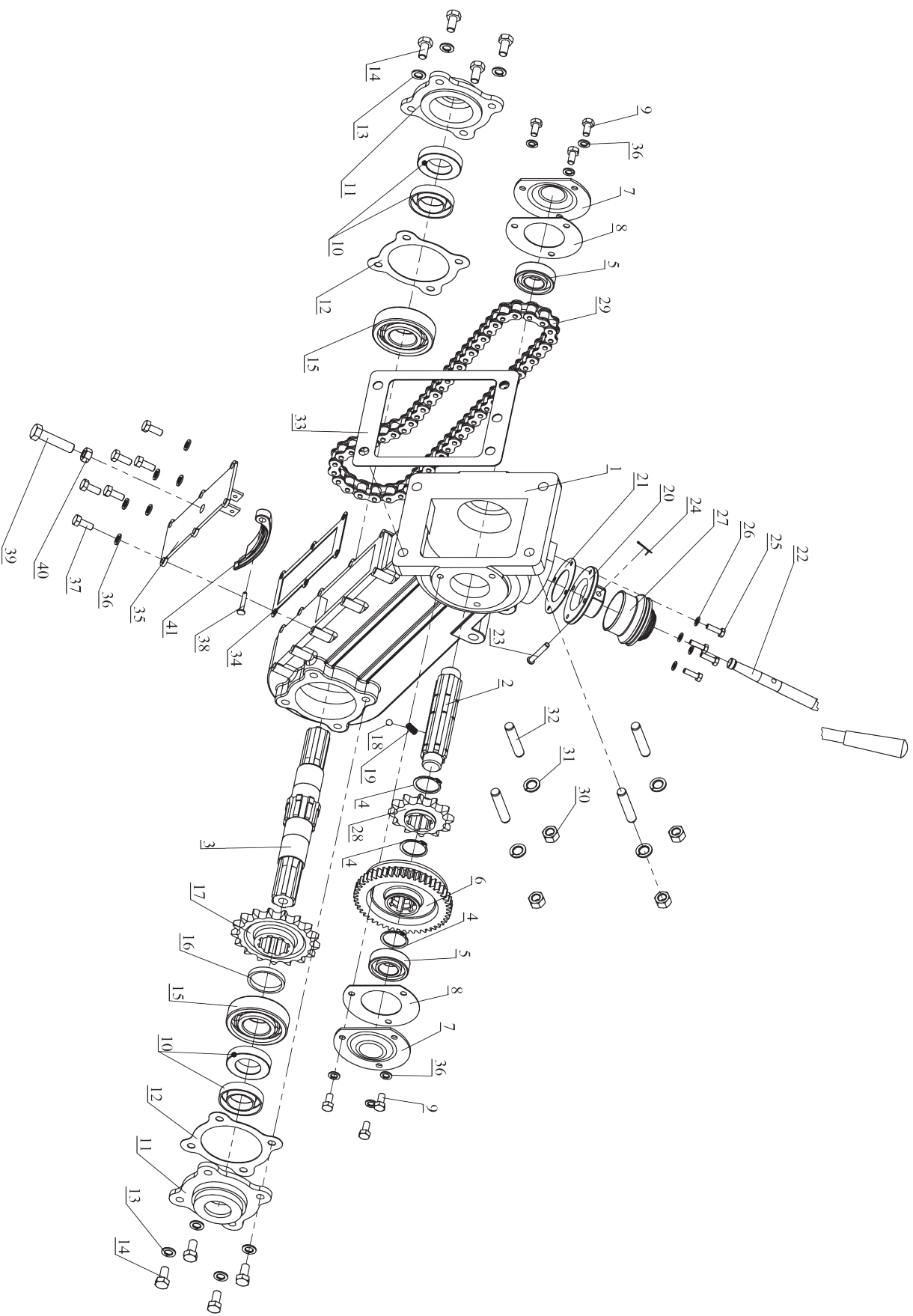
Рисунок 12. Комплектующие редуктора активной почвофрезы к тракторам и мотоблокам «Скаут» с шириной обработки 1000 мм.
