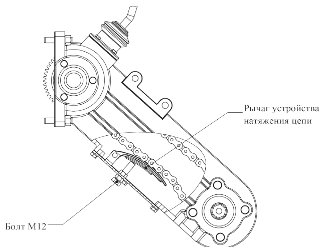
Рисунок 10. Устройство натяжения цепи.
