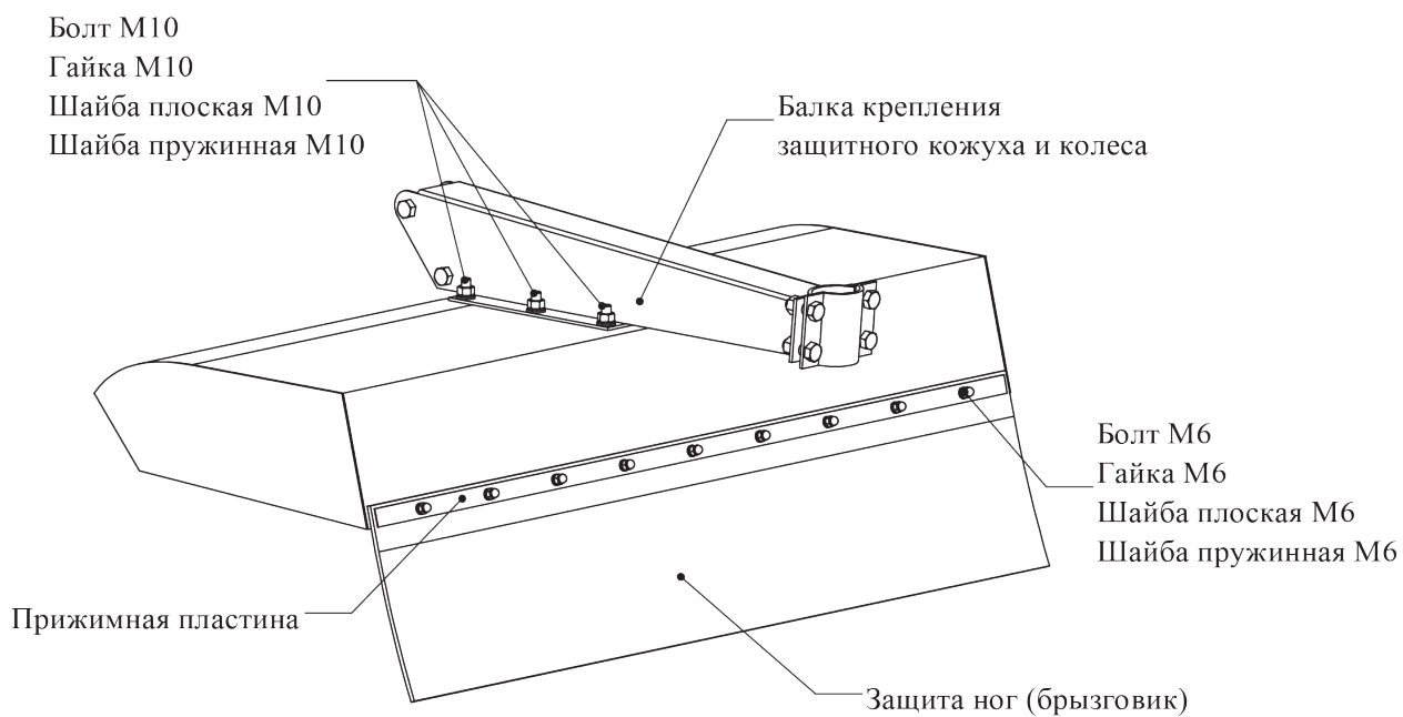
Рисунок 7. Сборка защитного кожуха на почвофрезе с шириной обработки 1000 мм.
